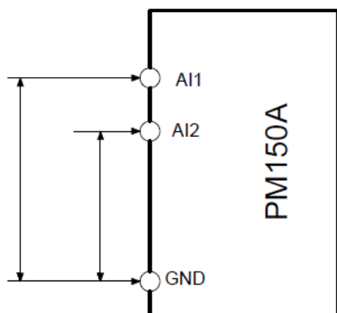
Рис. 6-2. Схема подключения аналогового входа при использовании внешнего источника питания
