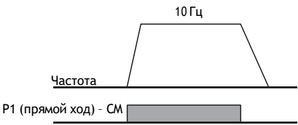
[Рабочая характеристика]
