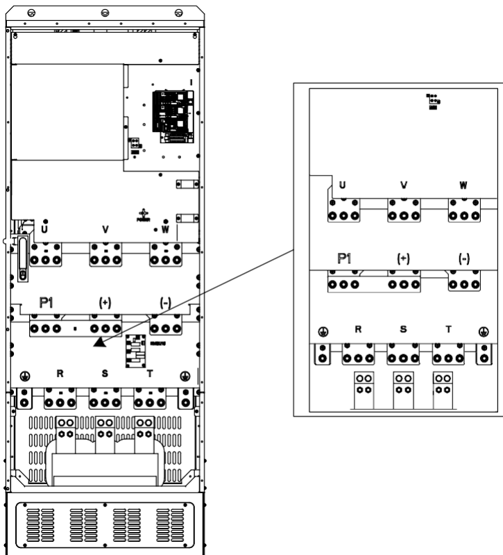
Рис 4.14 Клеммы силовых цепей ПЧ 355G/400P–500G
