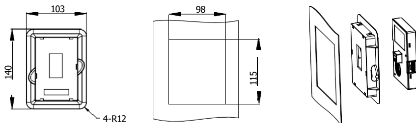
Кронштейн адаптера клавиатуры
