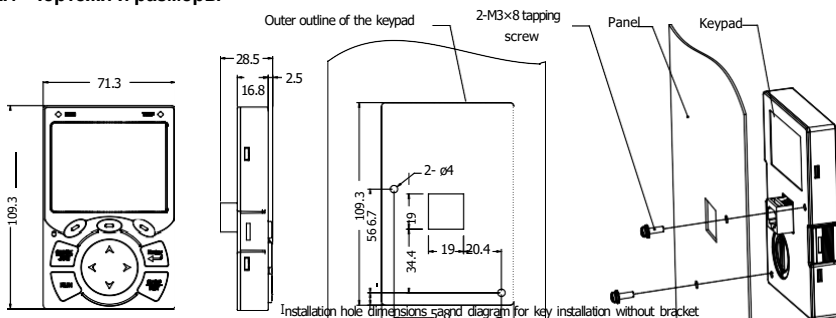
Рис 0.1 Размеры панели управления
