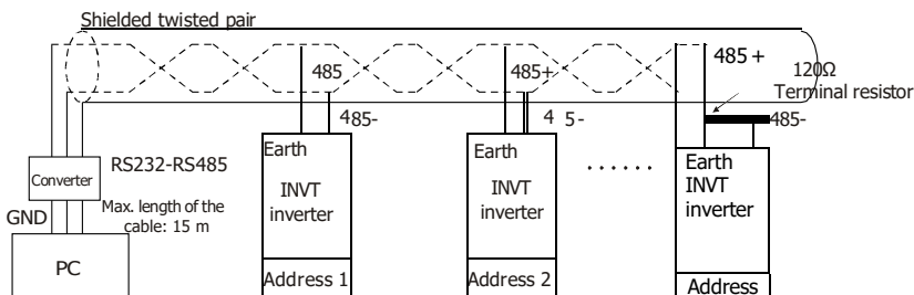
Рис 9.4 Практическая схема
