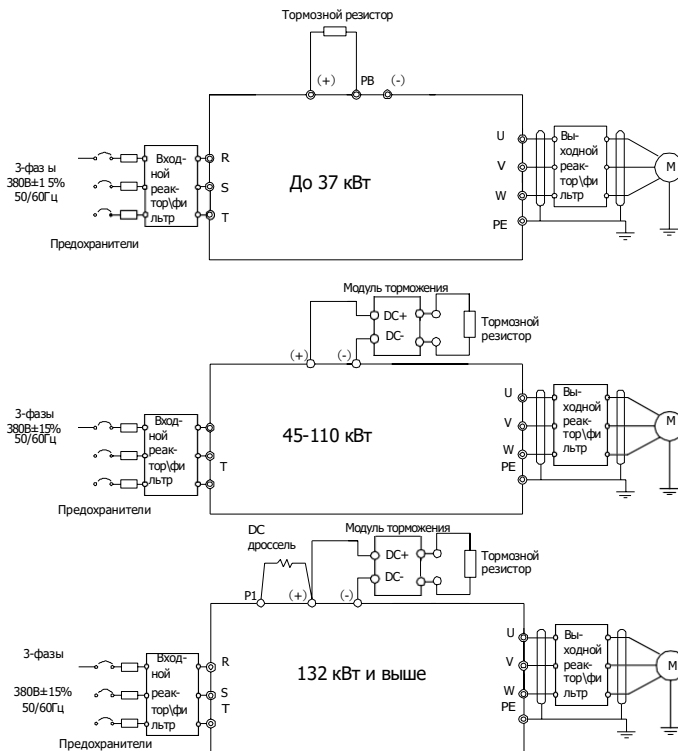
Рис 4.7 Схема подключения силовой цепи 380 В(-15%)–440 В(+10%)
