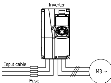
Рис 4.22 Подключение предохранителей
