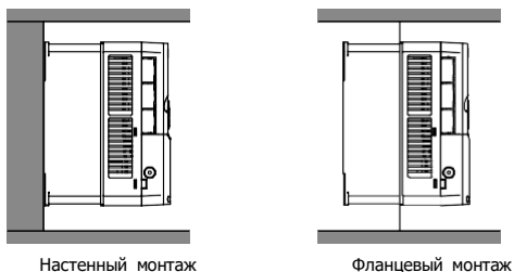
Рис 4.2 Способы установки
