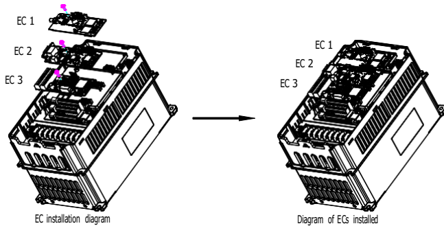
Рис 0.1 ПЧ 7,5 кВт или выше с установленными платами расширения
